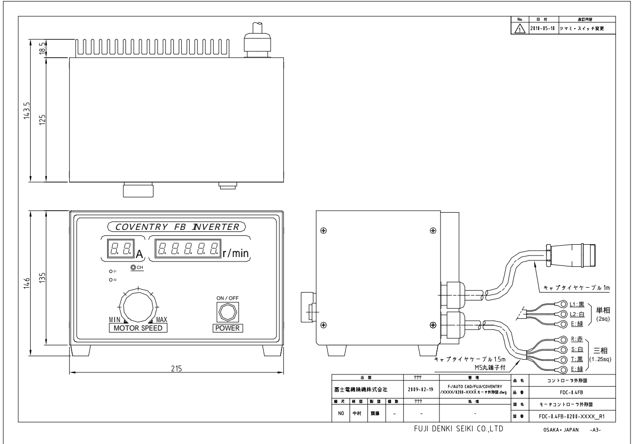
外形図
